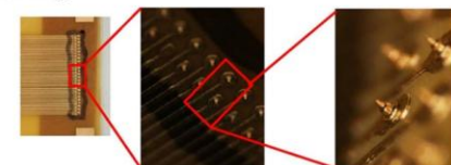
オス側 (Stud Bump)
