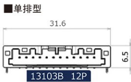
■ 基板侧连接器尺寸比较(单位:mm)
